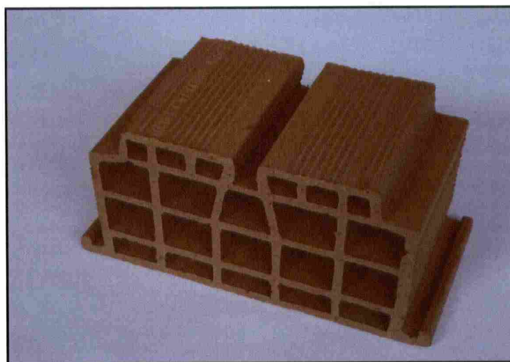
Blocco in laterizio denominato: PANNELLO 20/40 TG.20
